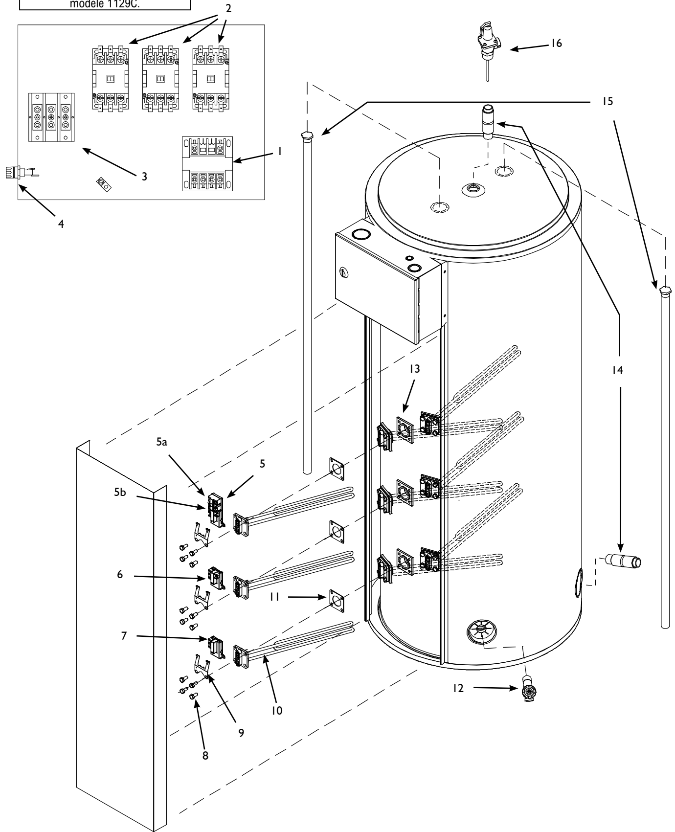
Disposition des pièces pour modèle 1129C.
