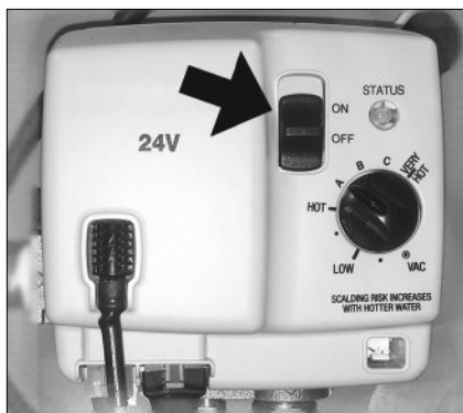
Figure 36 - Mettre l'interrupteur en position OFF (MARCHÉ).
