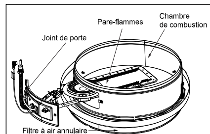
Figure 42 - Montage du brûleur.
