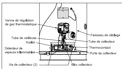
Figure 41 - Vue avant du chauffe-eau avec la porte extérieure retirée.
