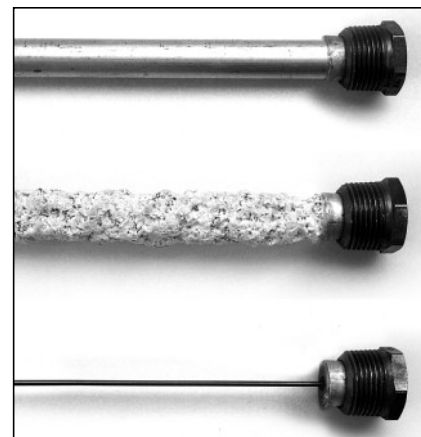
Figure 32 - Anodes neuve (haut), partiellement usée (milieu) et complètement usée (bas).
