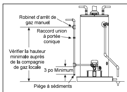
Figure 3 - Tuyauterie de gaz
