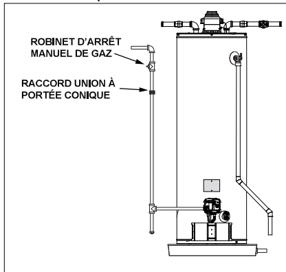
Figure 39 - Raccord union à portée conique
