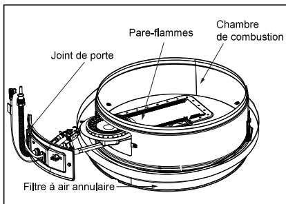
Figure 43 - Chambre de combustion
