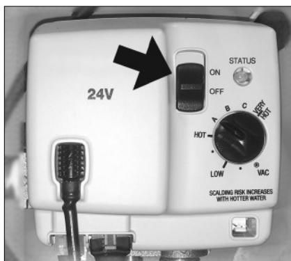
Figure 29 - Mettre l'interrupteur en position OFF (MARCHE).
