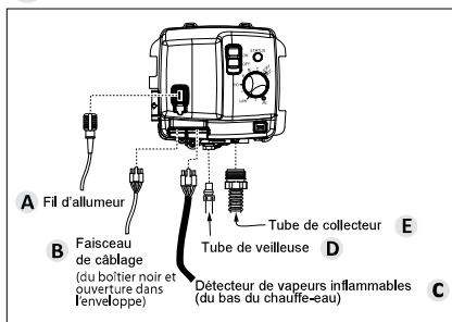
Figure 38 - Raccordements de la vanne de régulation de gaz
