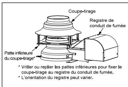
Figure 21 - Installer le coupe-tirage neuf.
