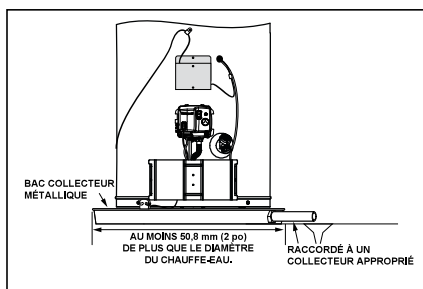
Figure 15 - Bac collecteur métallique raccordé à un écoulement.
