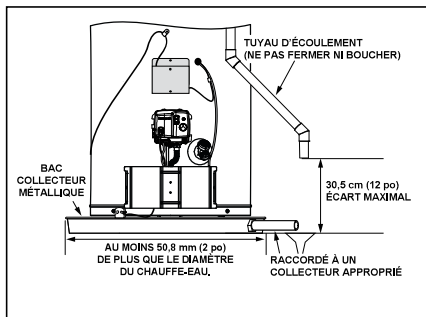
Figure 7 - Un bac collecteur métallique avec écoulement peut permettre de protéger le plancher des fuites et égouttements.
