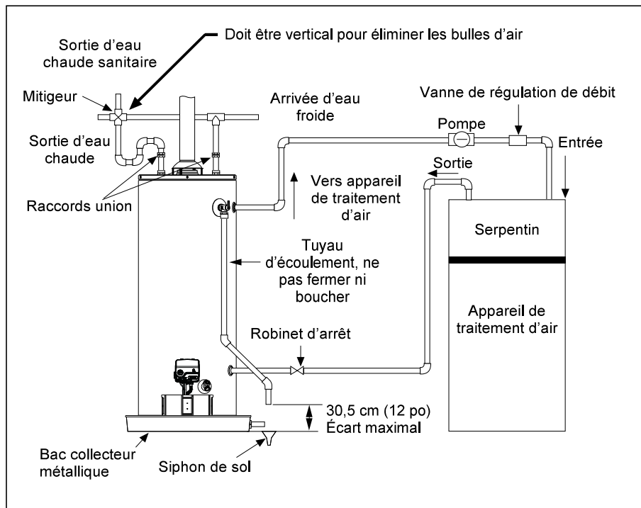
Figure 4 - Chauffage des locaux et de l'eau sanitaire (installation typique)
