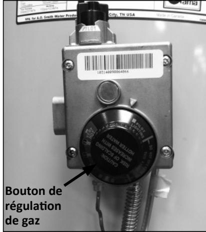
Figure 9 - Fermer la vanne de régulation de gaz/ température
