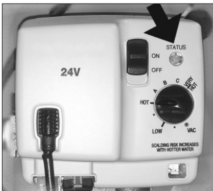
Figure 28 - Voyant d'état
