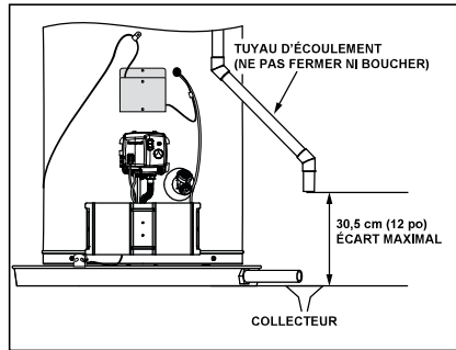
Figure 17 - Tuyau de la soupape de décharge à sécurité thermique (tuyau d'écoulement)
